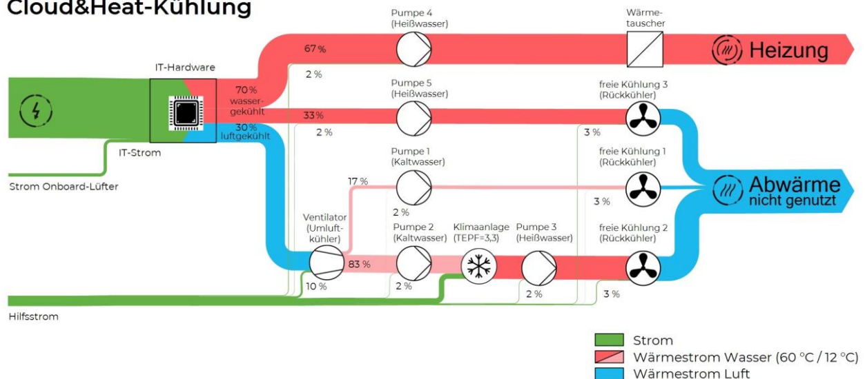
Abbildung 3: Energieflussdiagramme - klassische Luft- und Cloud&Heat-Kühlung im Vergleich
